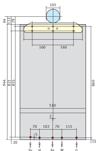
ISOFAST®
