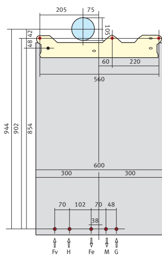
ISOTWIN
